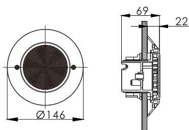
ELCOMP modelo sin nicho
