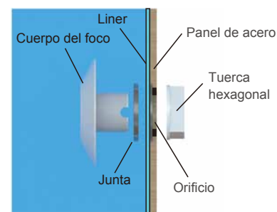
Piscina de paneles de acero con liner
