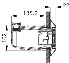
ELCOMP-N modelo con nicho
