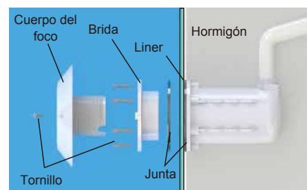
Piscina de hormigón con liner
